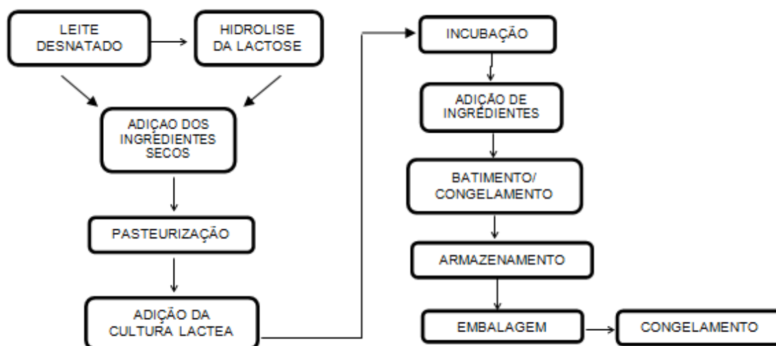
Figura 1. Fluxograma de processamento dos tratamentos de frozen yogurt elaborados com lactase e diferentes concentrações de inulina.
