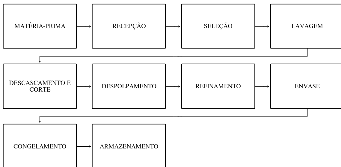
Figura 1 - Fluxograma das etapas de processamento de polpas de frutas congeladas realizadas na minifábrica.
